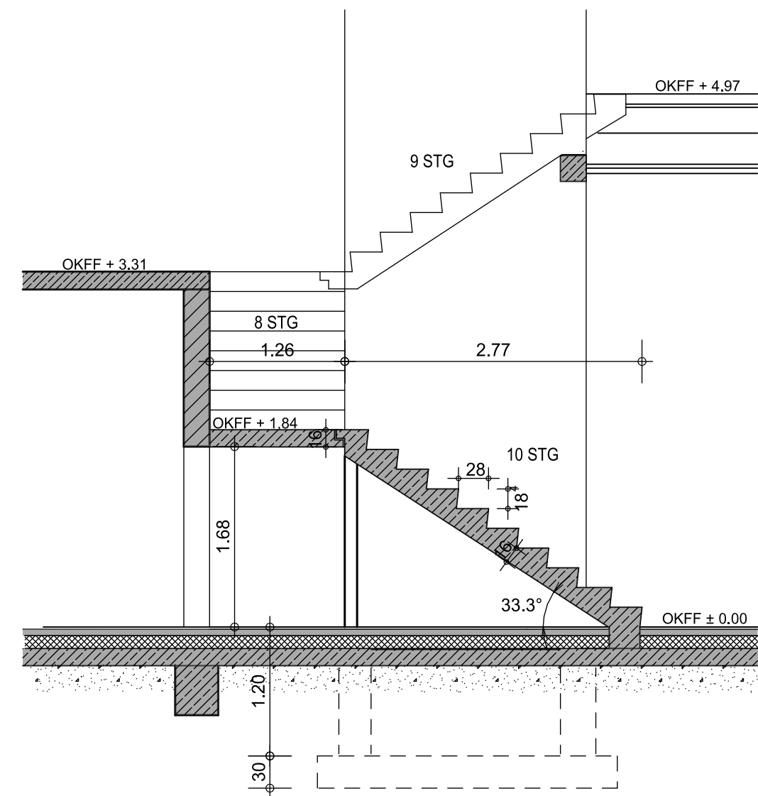
Schnitt Treppe 1:50
