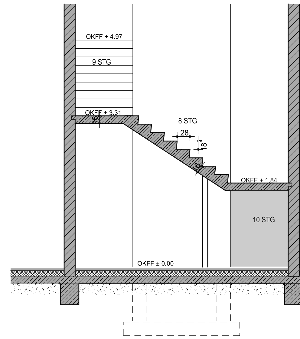
Schnitt Treppe 1:50
