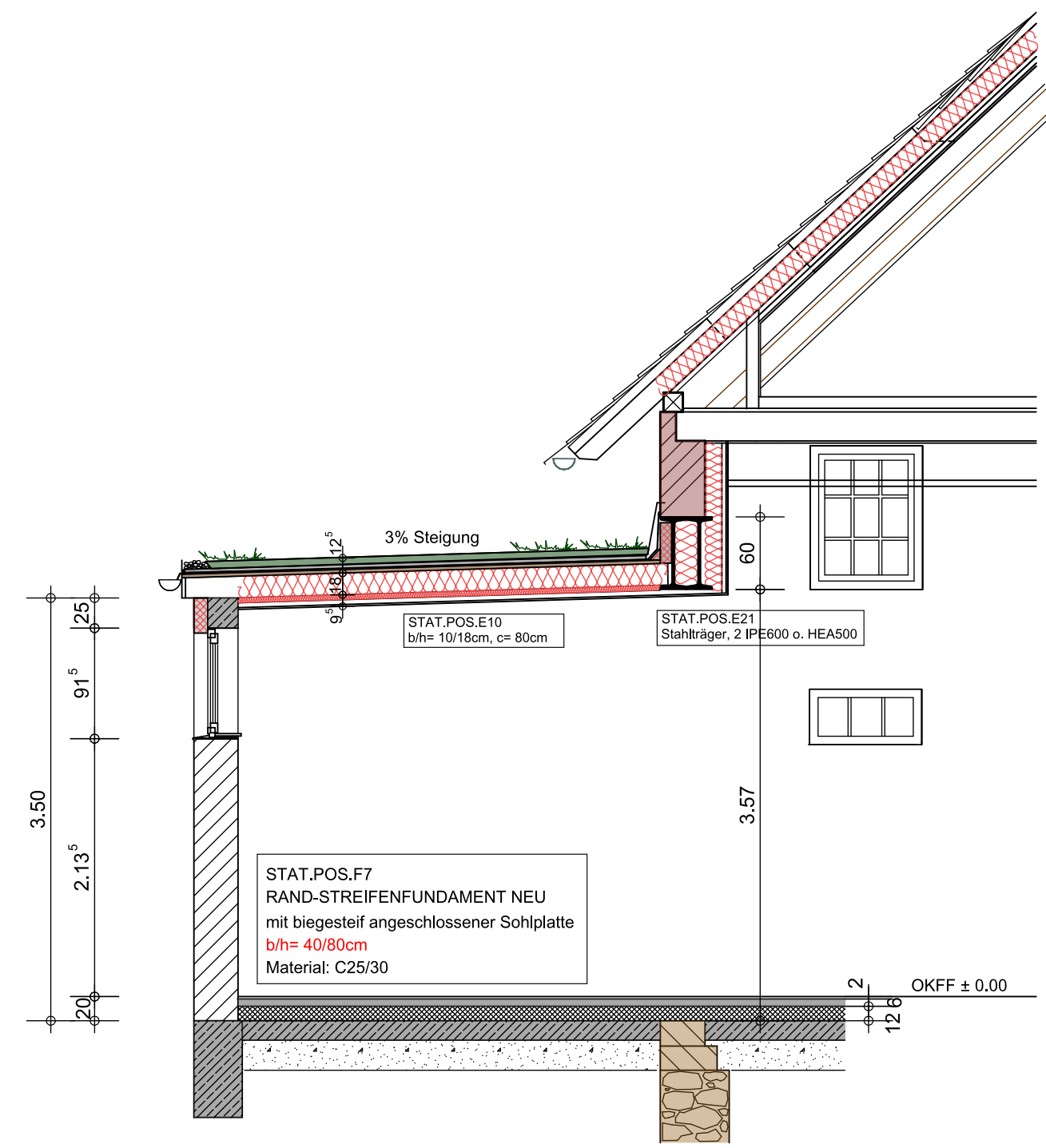
Schnitt Anbau 1:50
