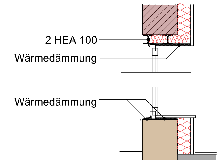
Fenster Clubraum Detail 1:25
